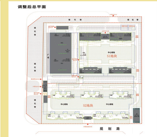
总平面布置图:1:750
