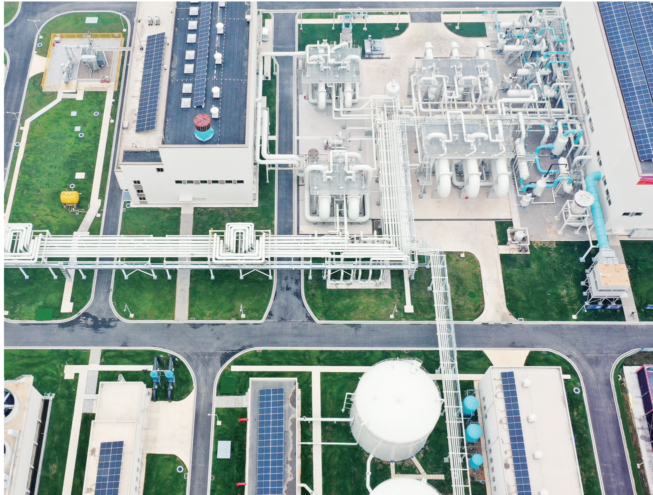
5月26日拍摄的江苏金坛盐穴压缩空气储能电站（无人机照片）。当日，江苏金坛盐穴压缩空气储能电站正式并网投运。盐穴压缩空气储能是指在电网负荷低谷期使用电能压缩空气，将其高压密封在地下的盐穴中，待电网负荷高峰期再释放压缩空气推动发电机发电，从而帮助电网错峰填谷。据介绍，该项目是我国首个盐穴压缩空气储能电站。
