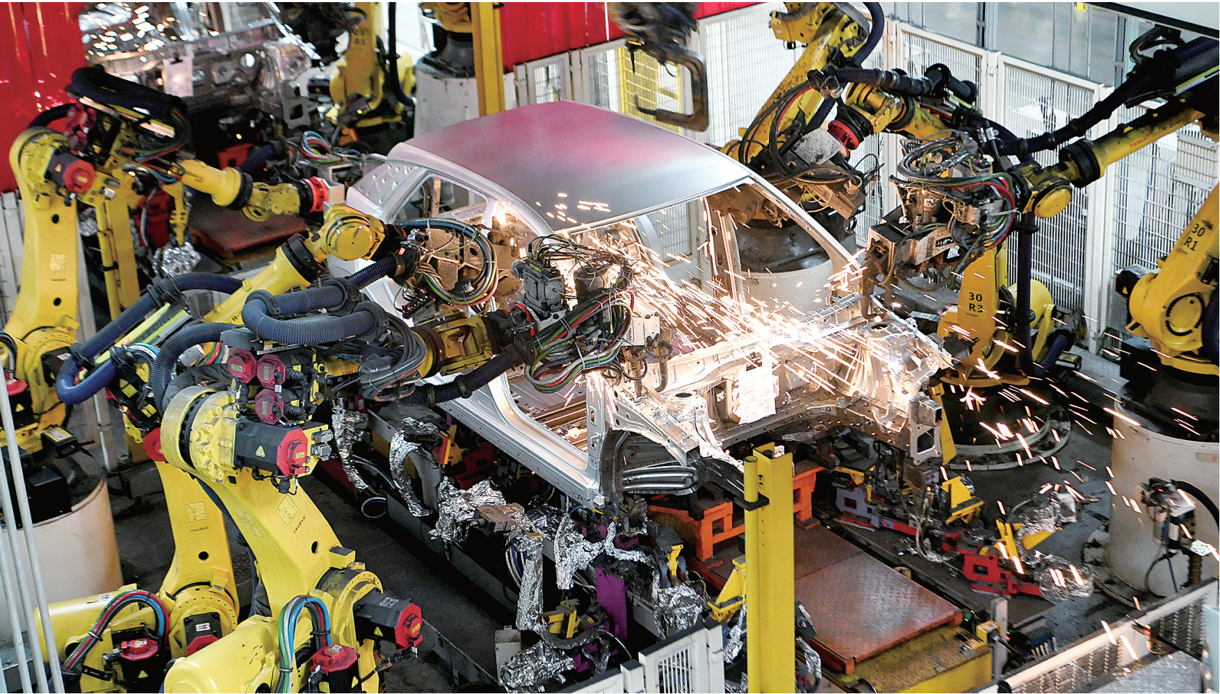
2月7日,机器人在上汽集团乘用车福建宁德基地车身车间生产线上作业。春节过后,各地企业开足马力忙生产,力争实现开门红。
