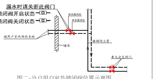
图二：分户用户室外锁闭阀位置示意图
