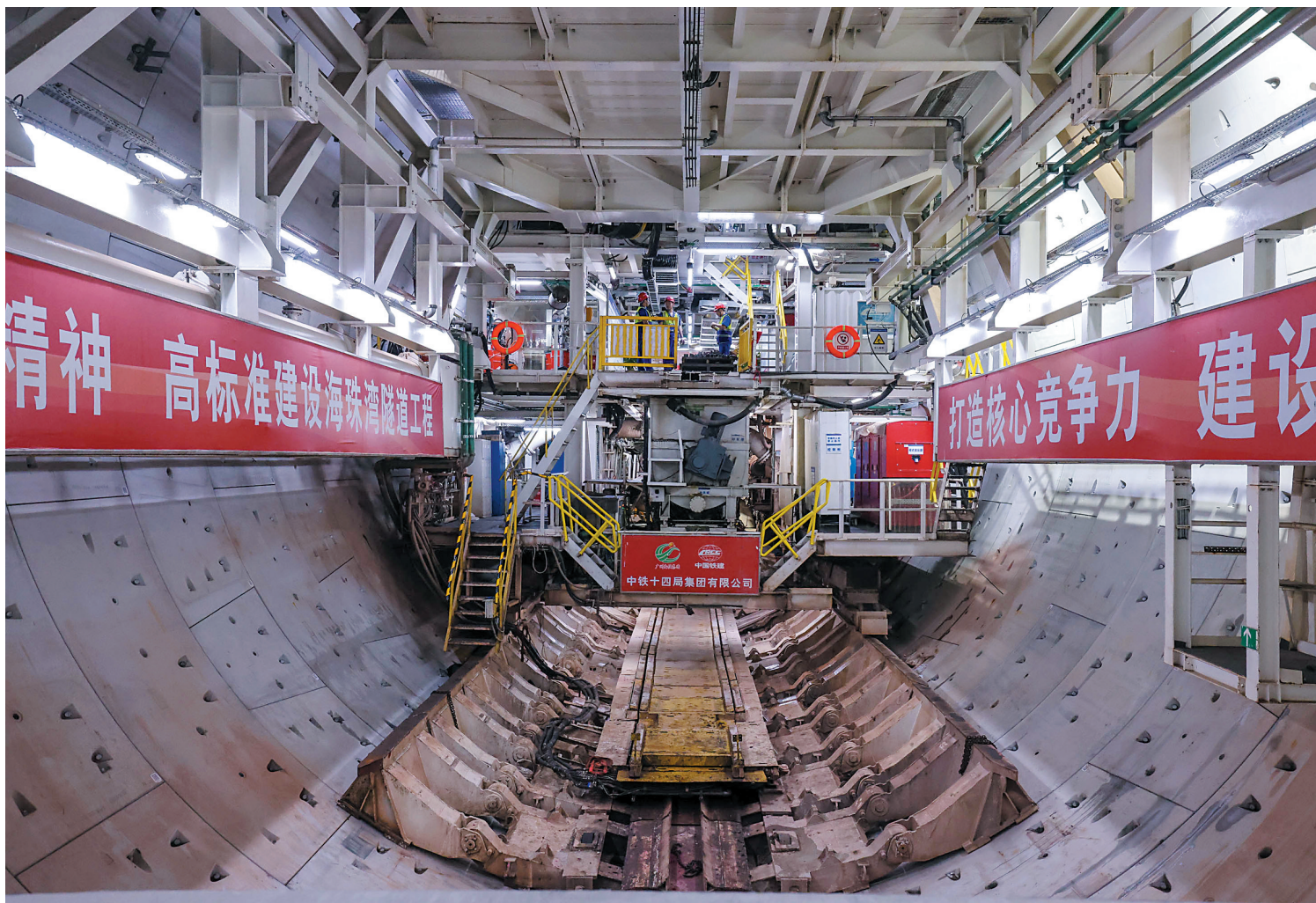
广州超大直径盾构机“双龙出洞”
