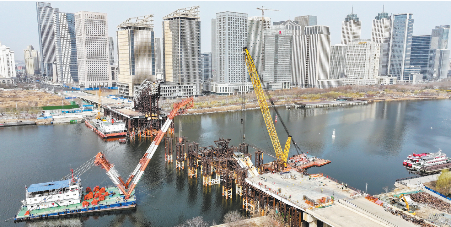
天津：‘海河’‘开启桥’建设稳步推进 这是三月十三日拍摄的位于天津市滨海新区的安阳桥。于新桥改建工程现场（无人机照片）。连日作业，位于天津市滨海新区的安阳桥，于新桥改建工程现场，各项作业稳步推进。根据设计方案，两桥均将改建为开启式桥梁。‘两桥’项目建成后，不仅将有效缓解该区域横跨海河的交通压力，还能为海河往来船只提供通航空间。 新华社记者 赵子硕摄
