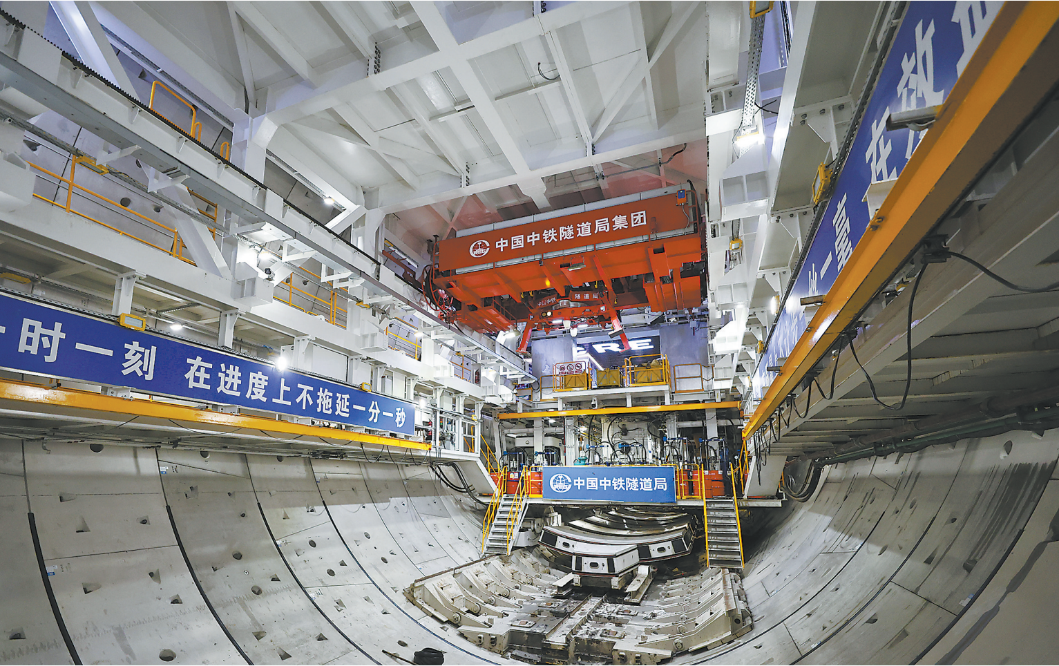
这是4月16日拍摄的“领航号”盾构机内的管片输送轨道(下)。 当日，我国自主研发的世界最大直径高铁盾构机——沪渝蓉高铁崇太长江隧道“领航号”在长江江底掘进至第2830环，累计掘进5660米，抵达长江江心。沪渝蓉高铁崇太长江隧道“领航号”盾构机刀盘直径15.4米，搭载智能掘进、智能拼装、超前地质预报等创新技术，以“有人值守、无人操作”的方式掘进。 新华社记者 方喆摄
