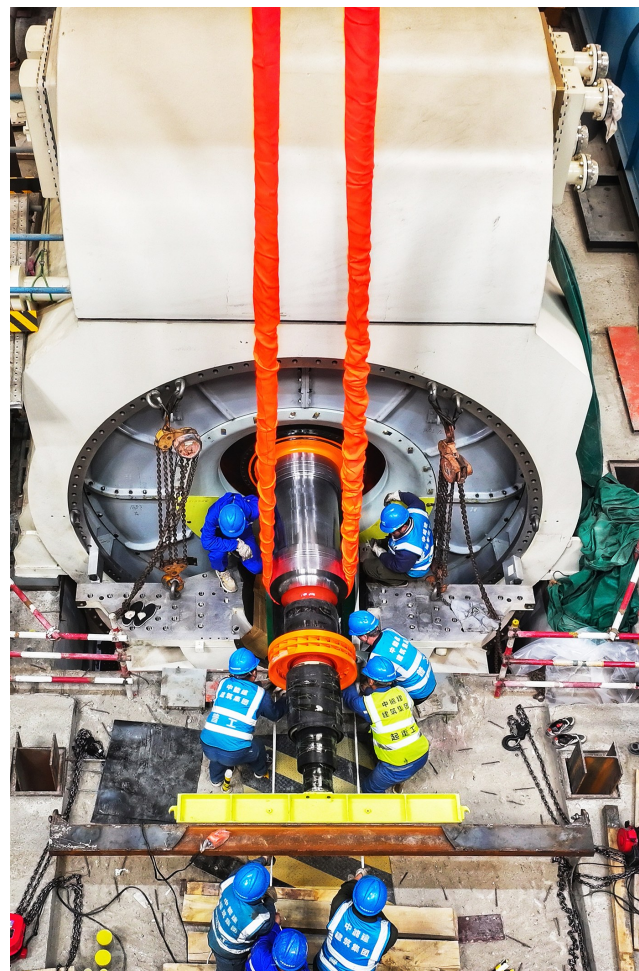
10月3日，国电电力大同湖东发电有限公司1号机组发电机转子穿装作业一次成功，标志着该机组大件全部就位。 此次穿装的转子由东方电气集团制造，采用“水—氢—氢”冷却技术，长15.04米、重96.6吨，对作业精度要求极高。作业中，工作人员采用“双行车协同吊装+电动葫芦精准推进”工艺，全程监测关键参数，历经5小时连续作业，转子平稳穿入定子，各项指标均符合标准。 本报记者 张占兵摄
